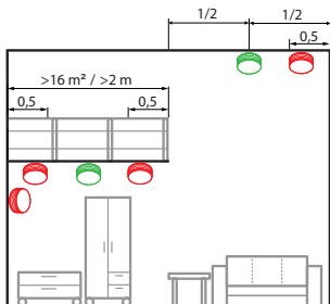
Abb. 7 Räume mit Podest oder Galerie
